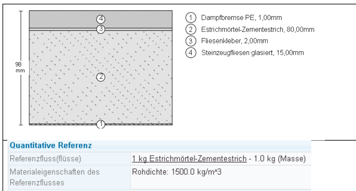
Abbildung 1: Grafische Darstellung Estrichmörtel-Zementestrich in eLCA bei Materialangaben Masse und Rohdichte
